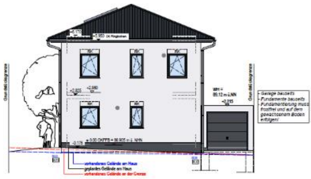
Ost-Ansicht
